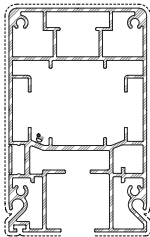
PQ501 Guida dim. 113x70 cm
