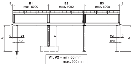
Vista frontale 3 moduli accoppiati
