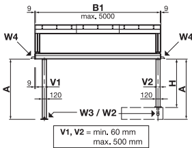
Vista frontale modulo singolo
