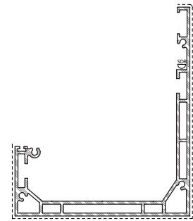
PQ502 Canale anteriore dim. 156x130 cm
